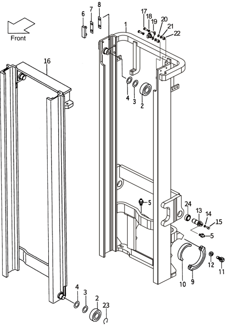
Fig.57 MAST [VM21A]
