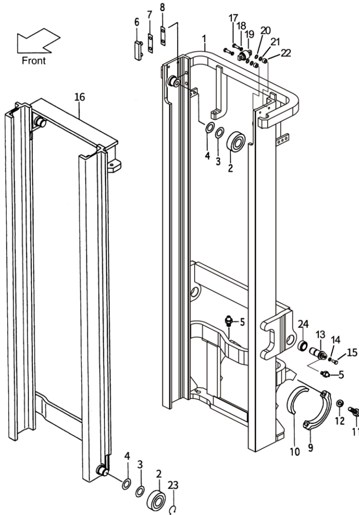
Fig.57 MAST [VM21A]
